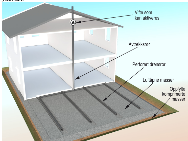
§ 13-5 Figur 1: Drensslanger under plate på grunn med et felles avtrekksrør som føres over terreng eller opp over bygningens yttertak.
