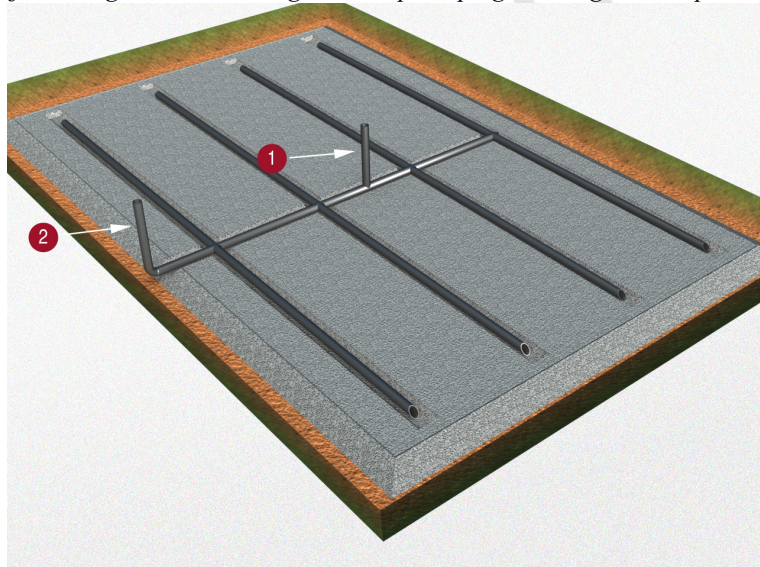
§ 13-5 Figur 2: Drensslanger under plate på grunn, lagt i det kapilærbrytende sjiktet.
