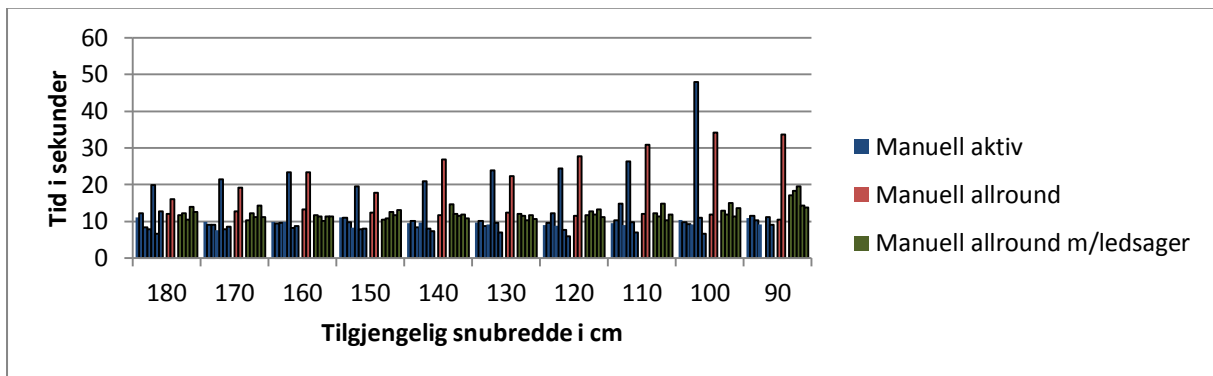
Figur 3.2.2-1: Testresultat for forsering av dør mot slagretningen for rullestoltypene manuell aktiv, manuell allround og ledsagerstyrt manuell allround
