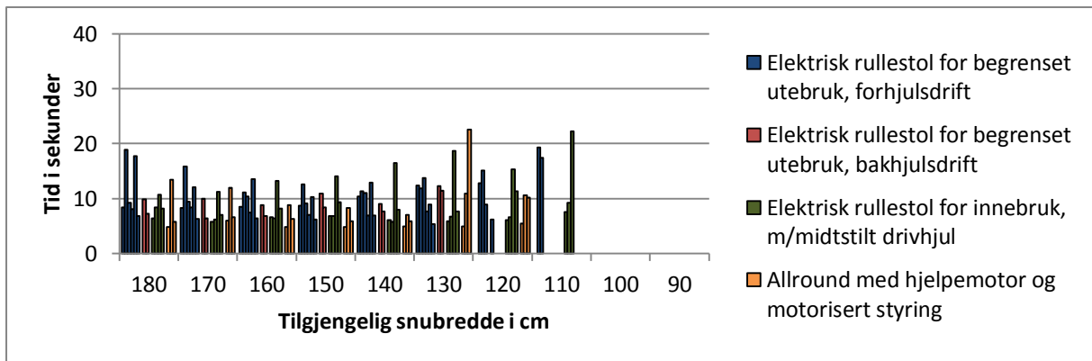
Figur 3.3.2-6: Testresultat for tidsforbruk ved test av snuareal. Rullestolrypene er elektrisk rullestol for begrenset utebruk, forhjulsdrift, elektrisk rullestol for begrenset utebruk, bakhjulsdrift, elektrisk rullestol for innebruk med midtstilt drivhjul og allround med hjelpemotor og motorisert styring
